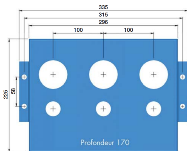
Dimensions de la carrosserie (en mm)
