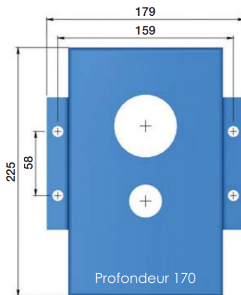
Dimensions de la carrosserie (en mm)
