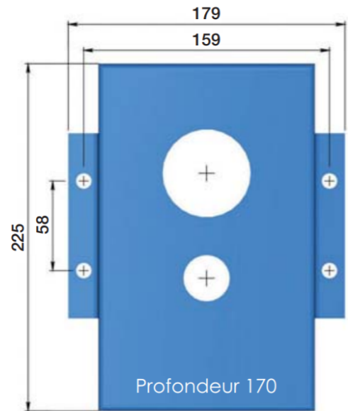
Dimensions de la carrosserie (en mm)
