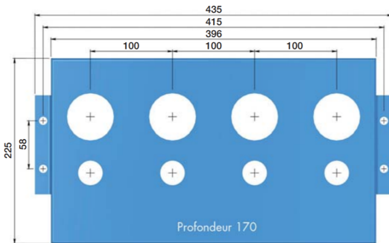
Dimensions de la carrosserie (en mm)
