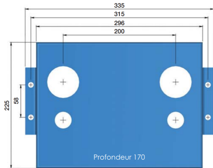
Dimensions de la carrosserie (en mm)
