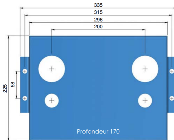
Dimensions de la carrosserie (en mm)
